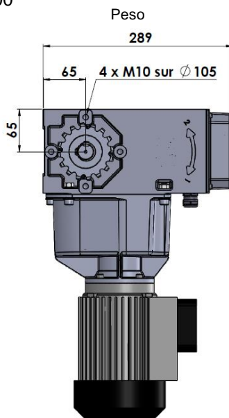
Accoppiamento a catena tubolare Ø32: MEC1100
