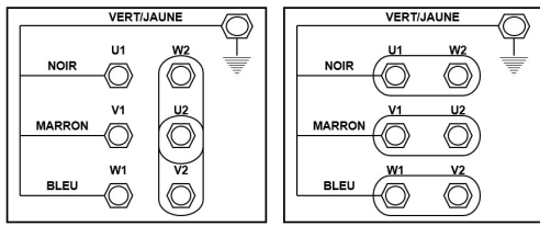
Raccordement de la plaque à bornes 400V TRI 230V TRI
